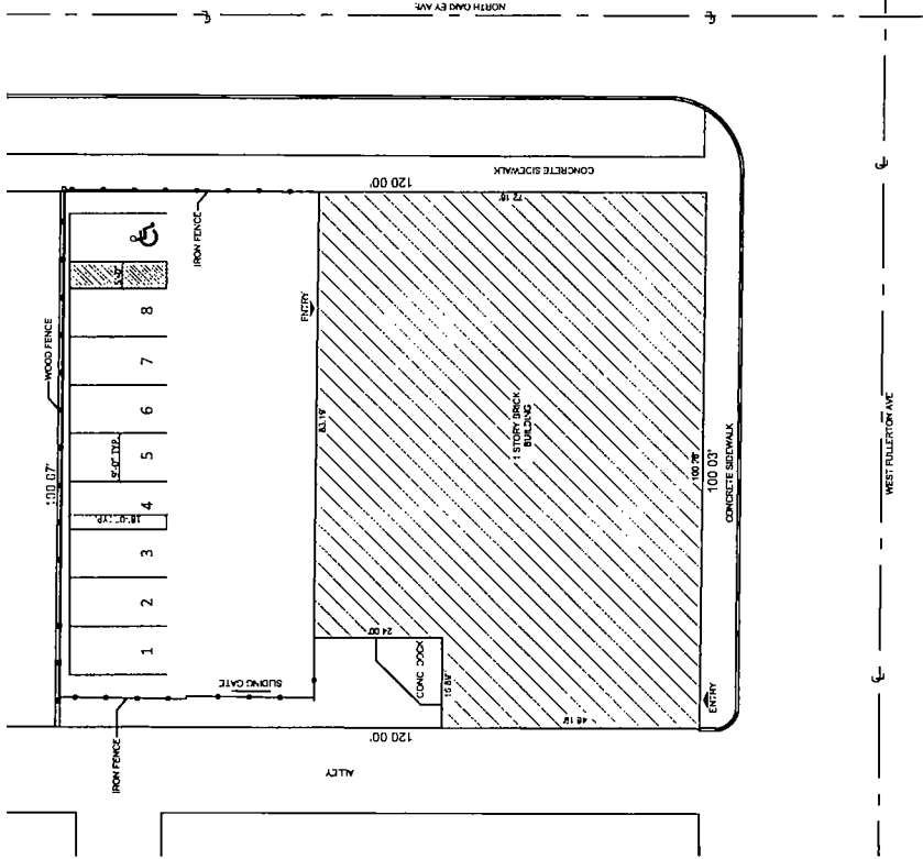
1. SITE PLAN A0 SCALE: 1"=12' 6"
